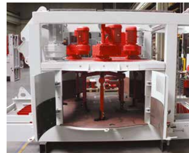
SM 3375 с доступом с обеих сторон для очистки и обслуживания
